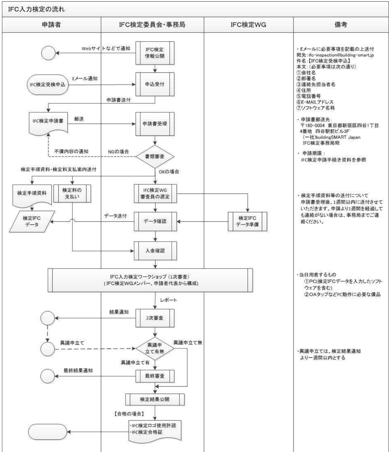
図-2 IFC 入力検定の流れ
